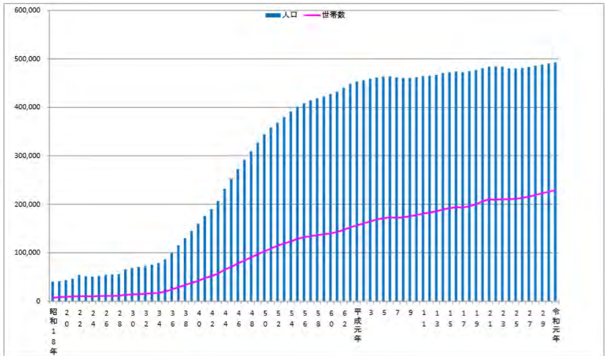
図 6-1-1 人口推移
