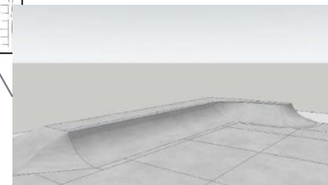
クォーターパイプ① (高さ1.0 m、長さ15.7 m)
