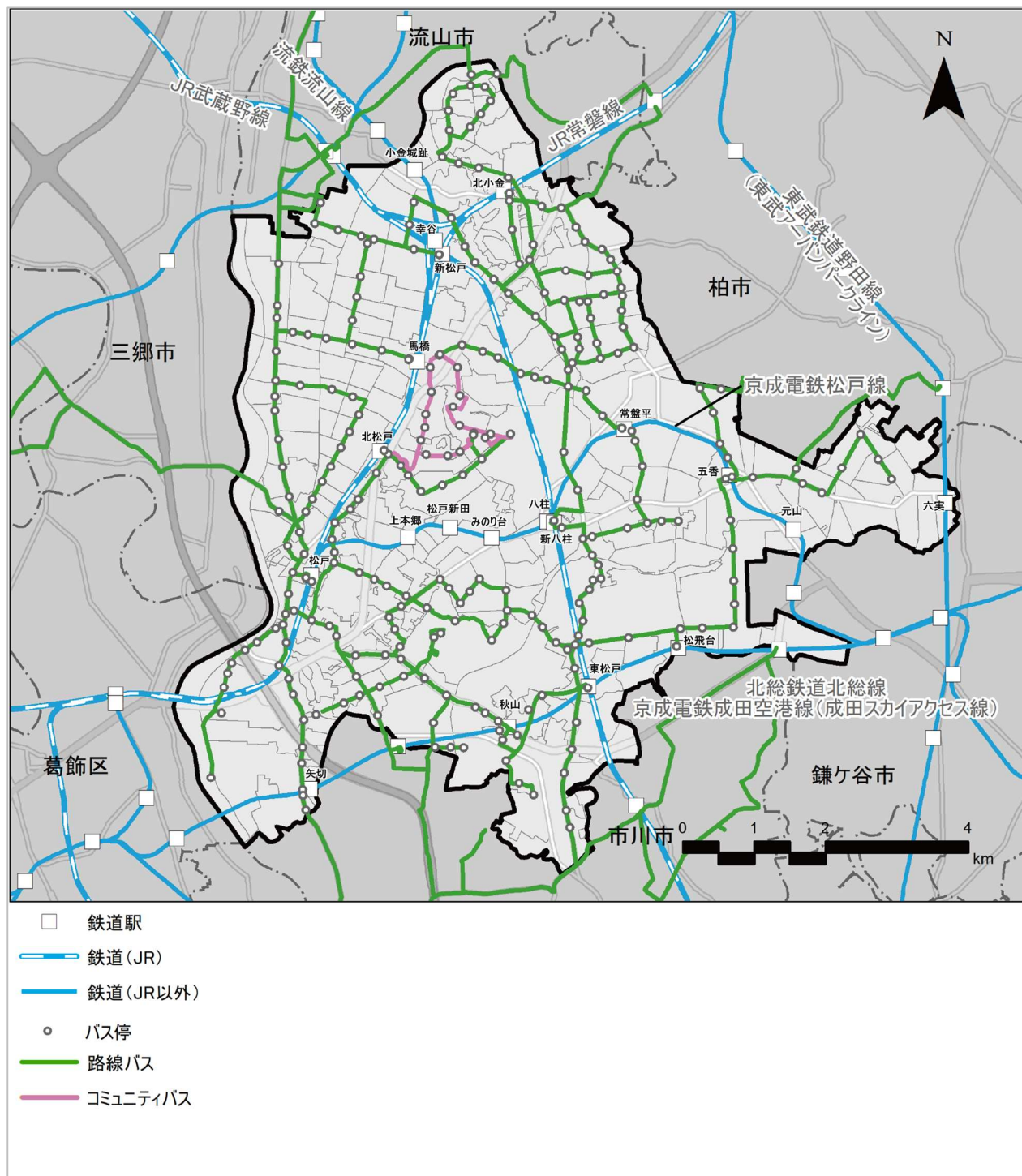
鉄道・バスの運行ネットワーク
