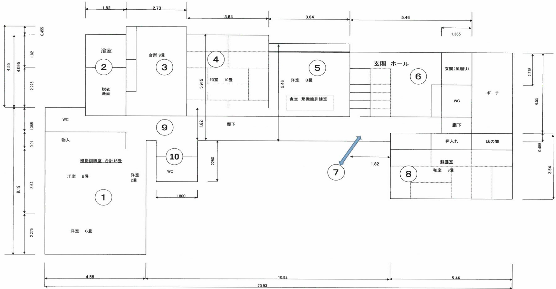
1階 平面図 求積図
