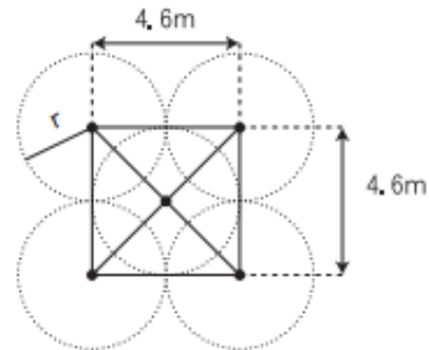
(散水密度が低下しないようにした千鳥型配置の例)
