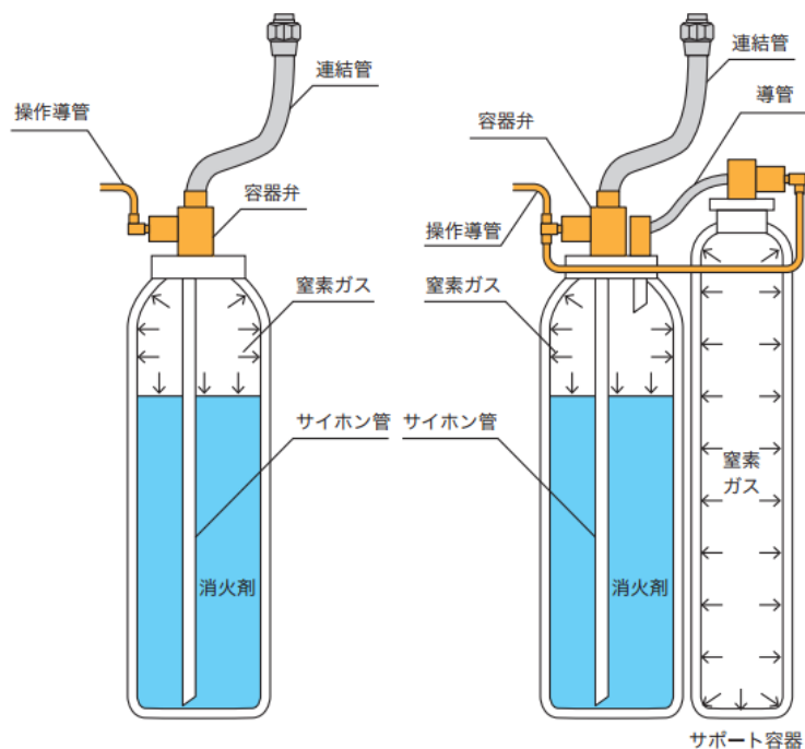
（参考）蓄圧式の貯蔵容器
