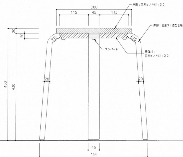
A-A 側断面図
