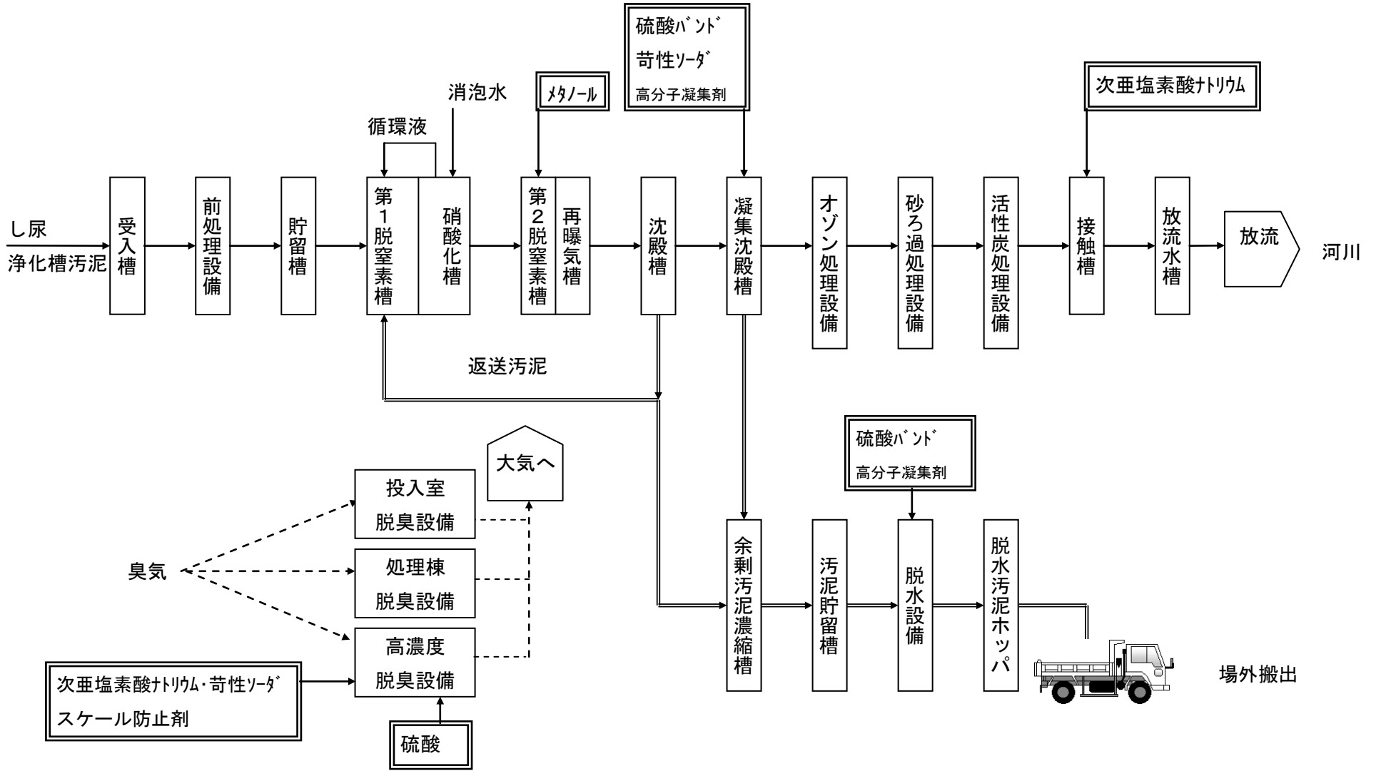
東部クリーンセンター処理工程概要図 (二重枠内が薬剤)
