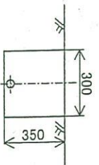
掘削断面図 (人力掘削・発生土埋め戻し)
