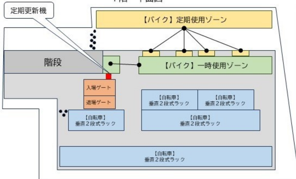
1階 平面図
