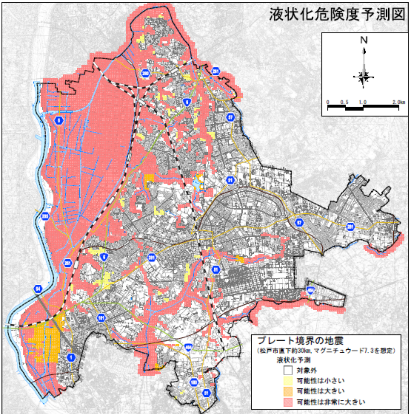
プレート境界の地震による液状化予測 (松戸市直下約30km, マグニチュード7.3)
