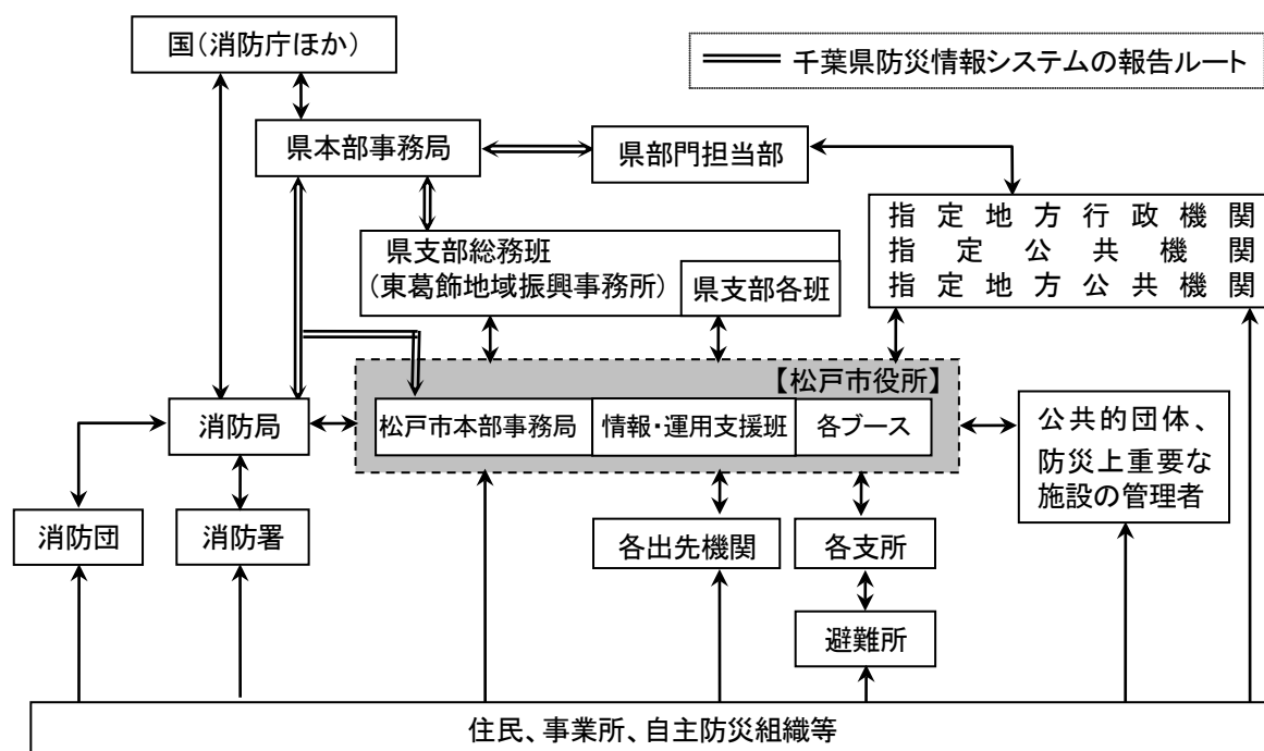
＜連絡系統図＞
