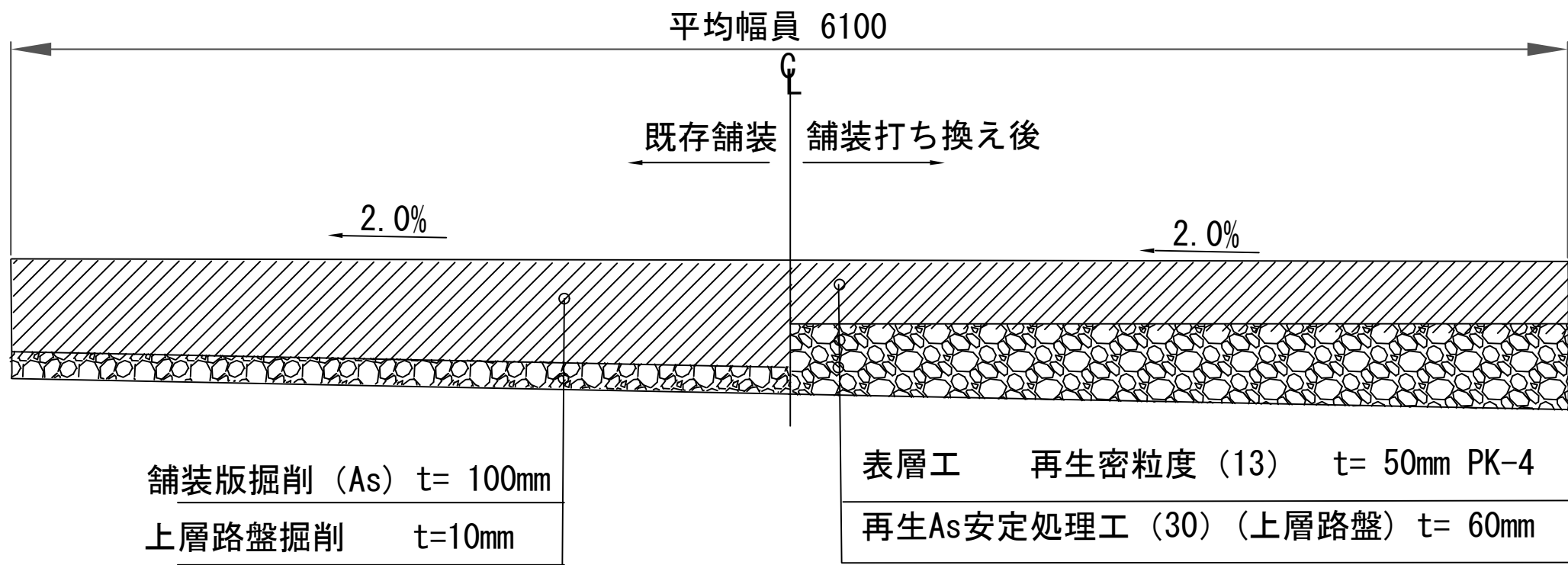
1区間 標準横断面図
