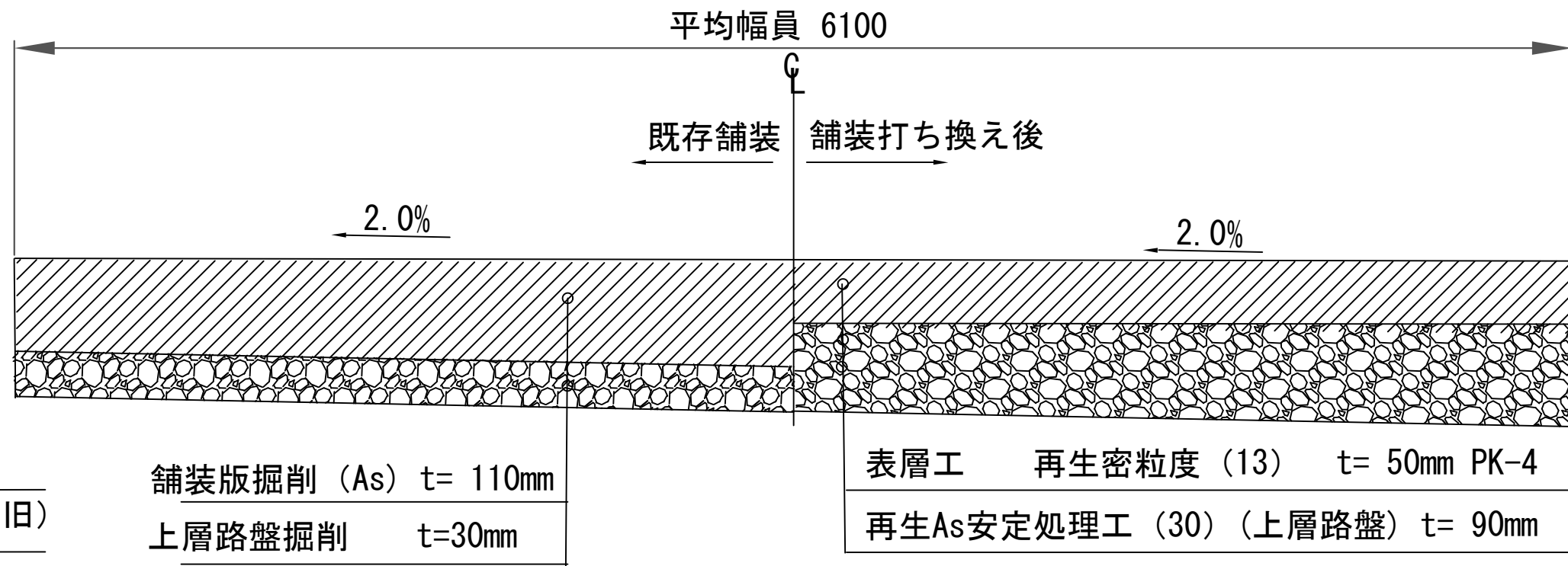
2区間 標準横断面図
