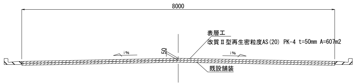
市道4地区598号 標準断面図
