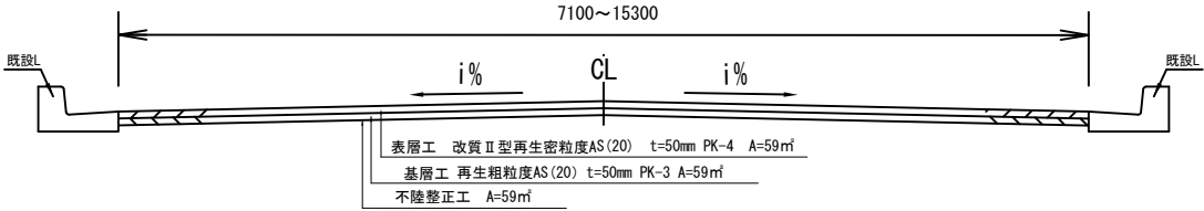
主要幹線1級市道19号 標準断面図
