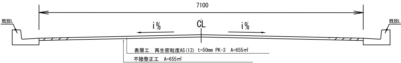
市道4地区71号 標準断面図
