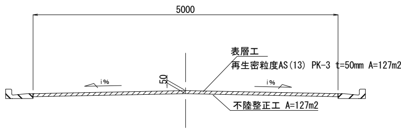
市道4地区263号 標準断面図
