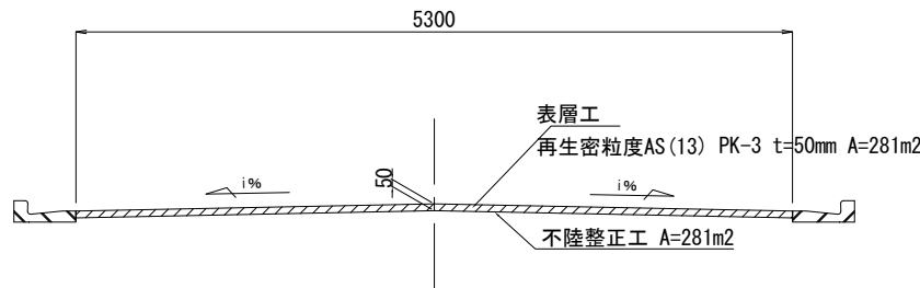
市道4地区190号 標準断面図
