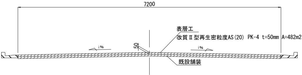
市道4地区158号 標準断面図
