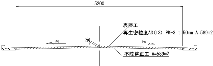
市道4地区156号 標準断面図
