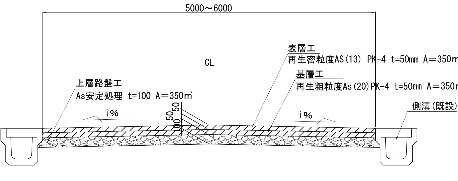
計画標準横断図 S = 1/20
