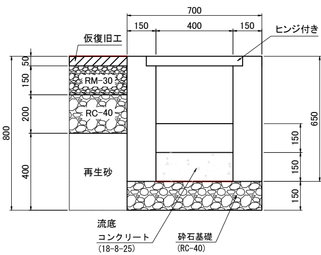
集水ます (400×400×650)
