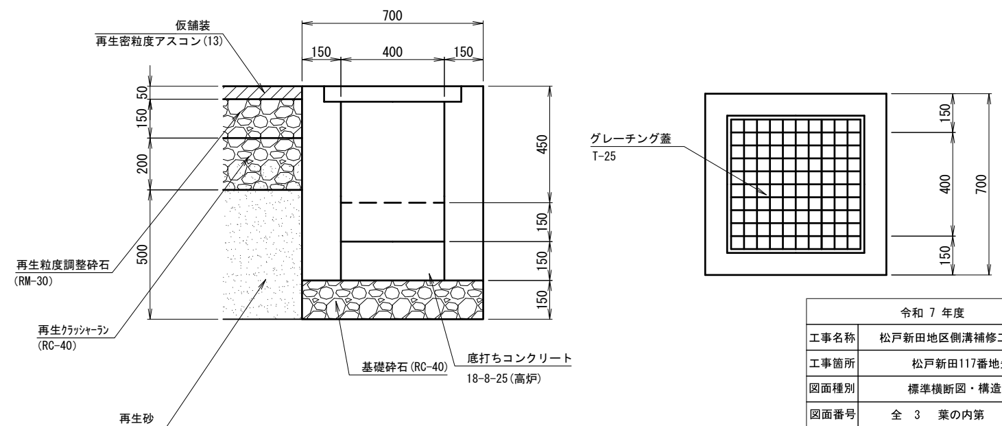
集水ます (400×400×750)
