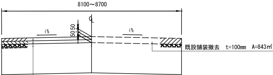
標準横断図 S=1/100
