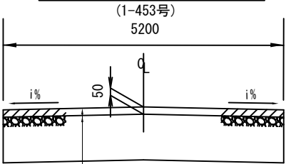
標準横断図 S=1/100
