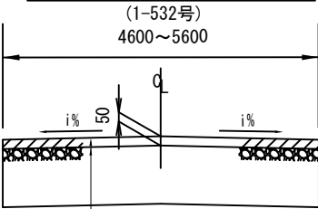
標準横断図 S=1/100
