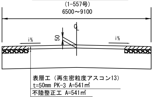
標準横断図 S=1/100
