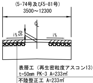
標準横断図 S=1/100
