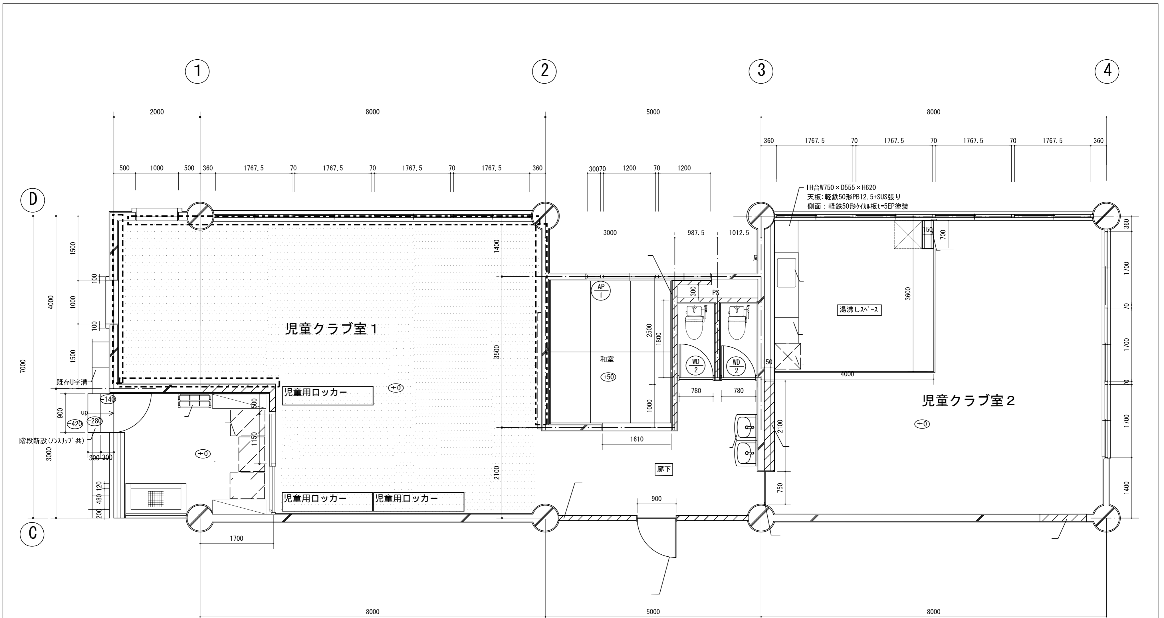
平面図 S=1/100
