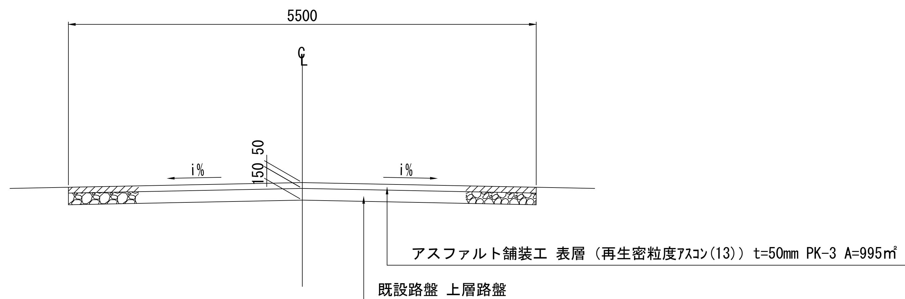
標準横断面図 S=1/20
