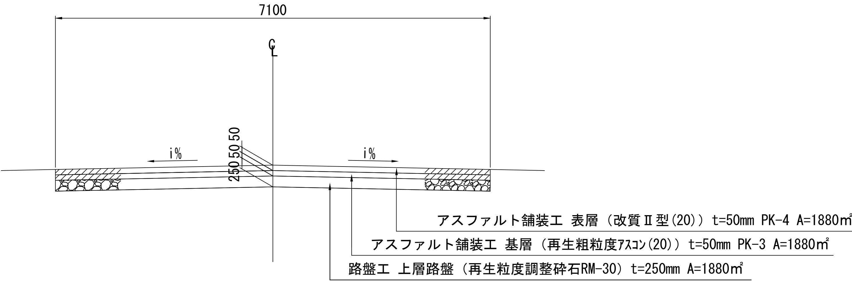
標準横断図 S=1/20
