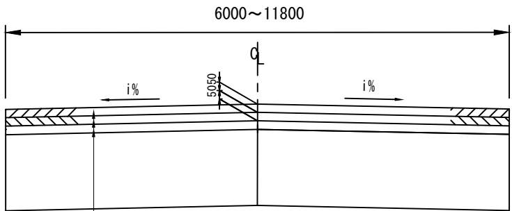
標準横断図 S=1/20
