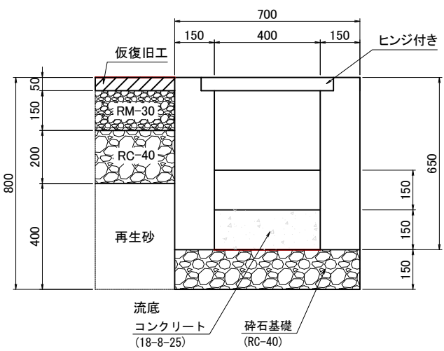
集水ます (400×400×650)
