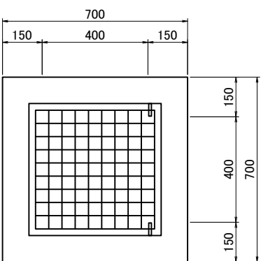
グレーチング (T-25)
