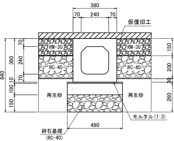
横断暗渠（240*240）
