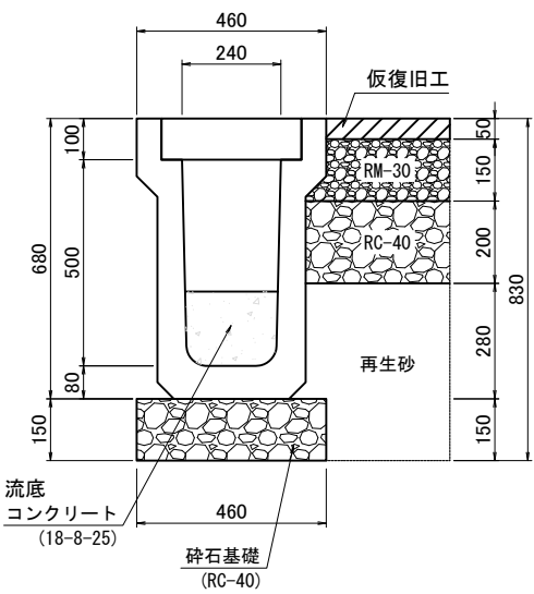
千葉県型側溝 (240*500)
