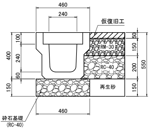
千葉県型側溝（240*240）
