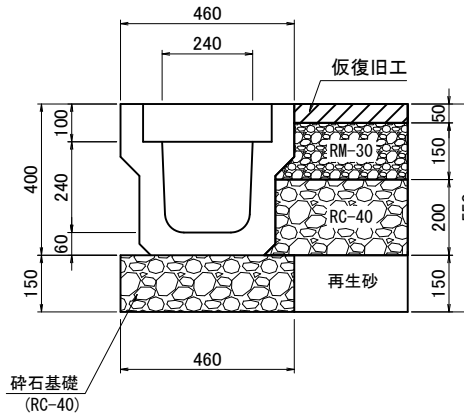
千葉県型側溝 (240*240)
