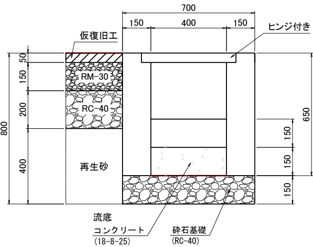
集水ます（400×400×650）
