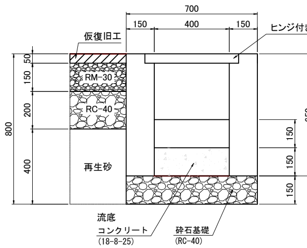
集水ます (400×400×650)
