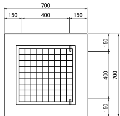
グレーチング (T-25)
