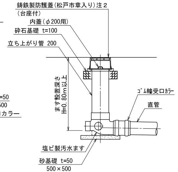
(取付管布設標準図)
