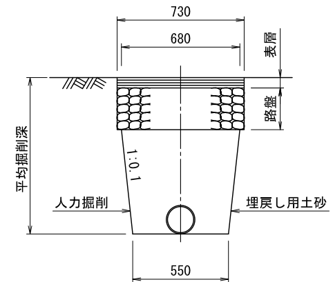
(取付管布設標準図)
