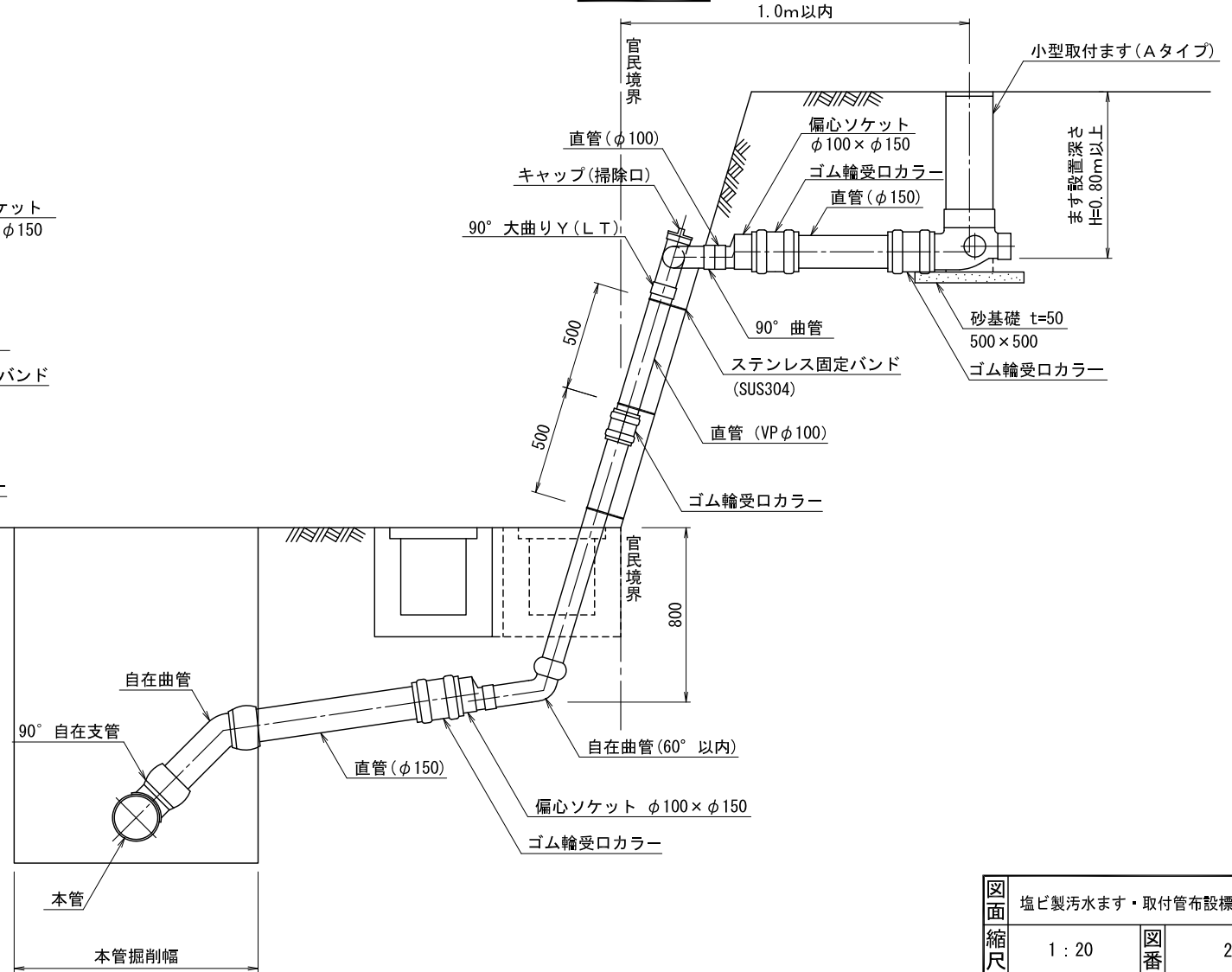
側面図
