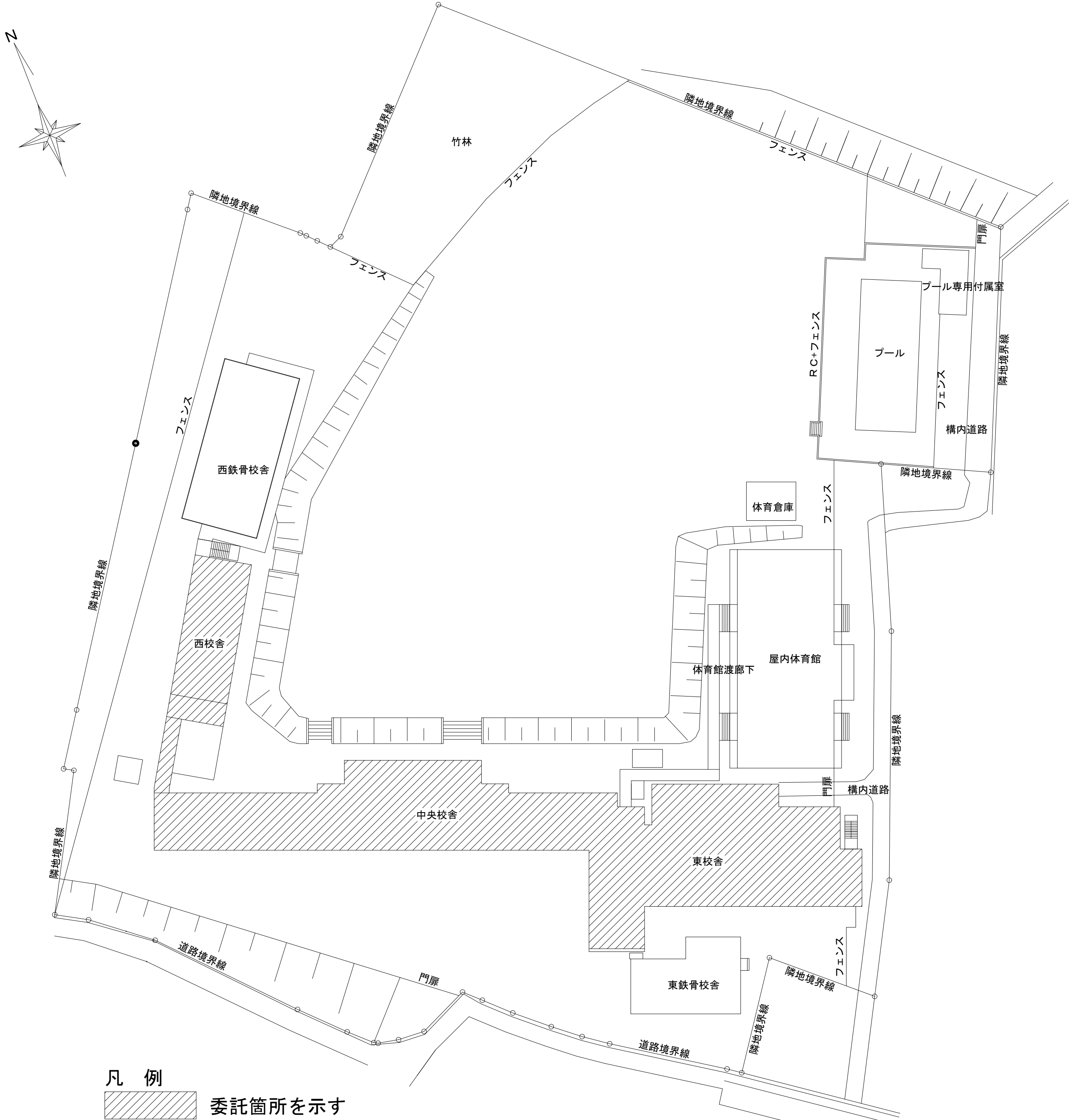
配置図 S = 1 : 500
