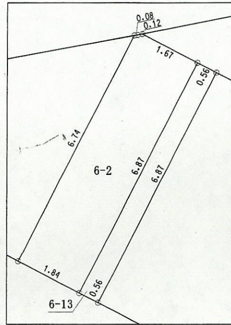
尺度=1/100
