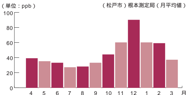
窒素酸化物の月別変化(平成15年度)
