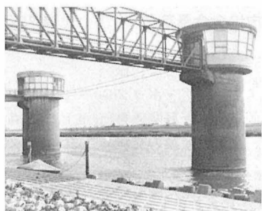
栗山浄水場の取水口、このすぐ上流には赤坂樋門が
