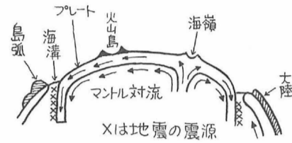
図1 プレートが生成され、消失する様子
