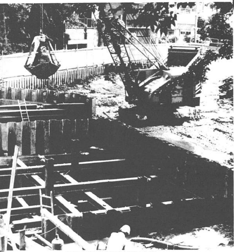
急ピツチで進む貯留池工事(小金きよヶ丘)
